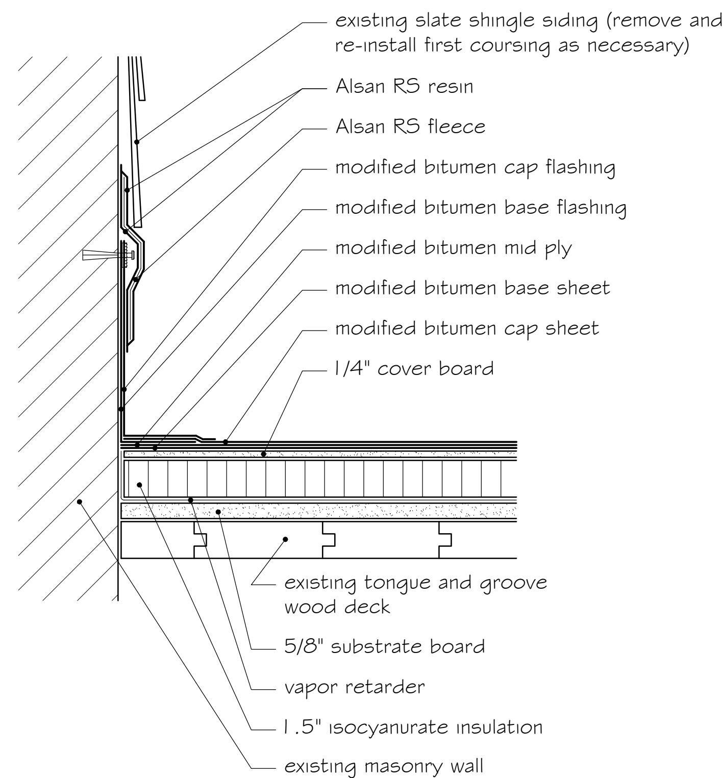
4 ROOF HATCH - AREA 29 SCALE: 1" = 4"
