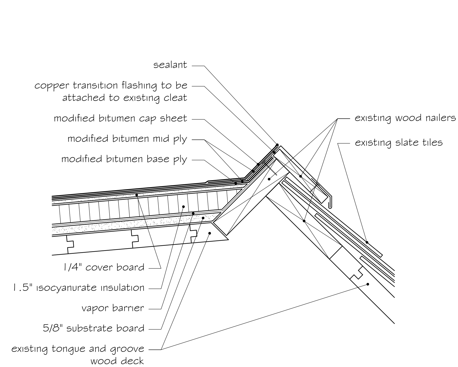
1 PERIMETER EDGE - AREA 29 SCALE: 1" = 4"
