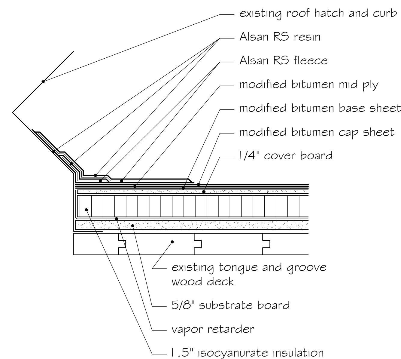
5 ROOF HATCH - AREA 29 SCALE: 1" = 4"
